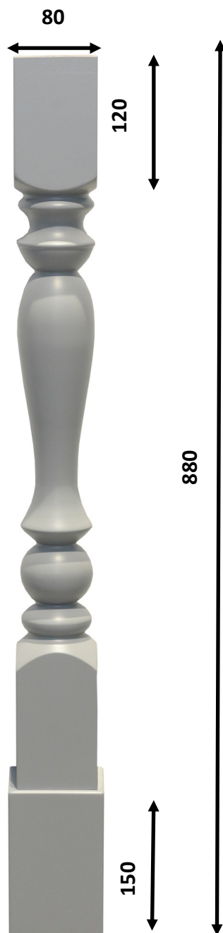
NOGA TOCZONA
